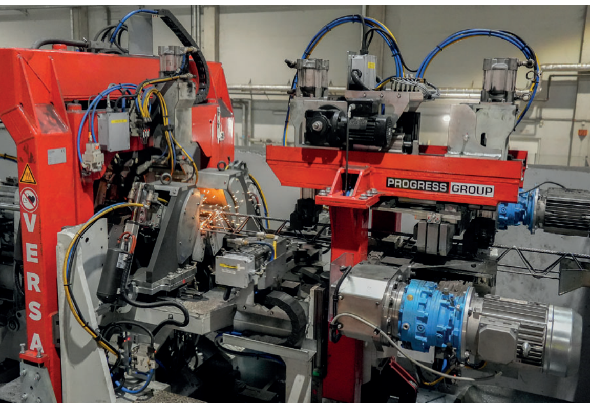
Новая машина для сварки решетчатых балок Versa для гибкого производства решетчатых балок с бухты
